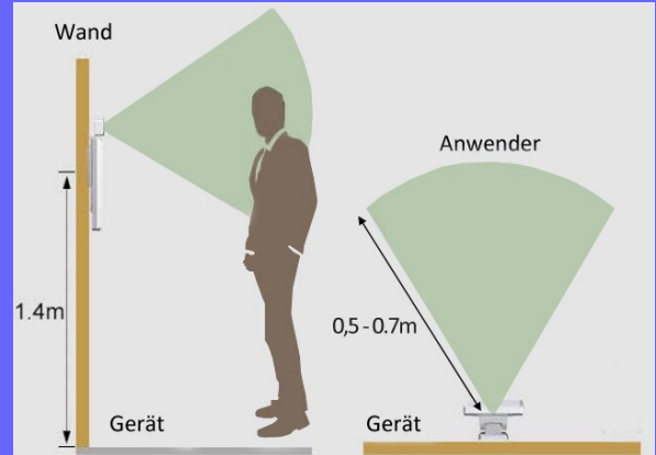
Messwinkel und Montagempfehlung
